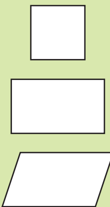
Parallelogramm
