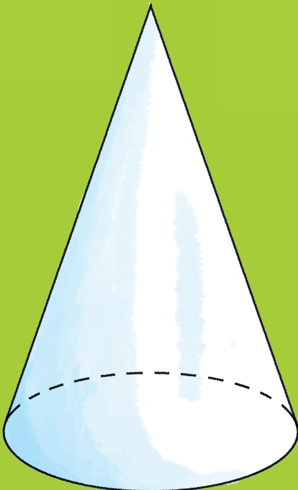
Kegel
