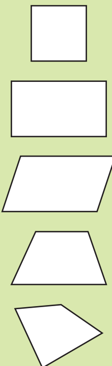
Viereck
