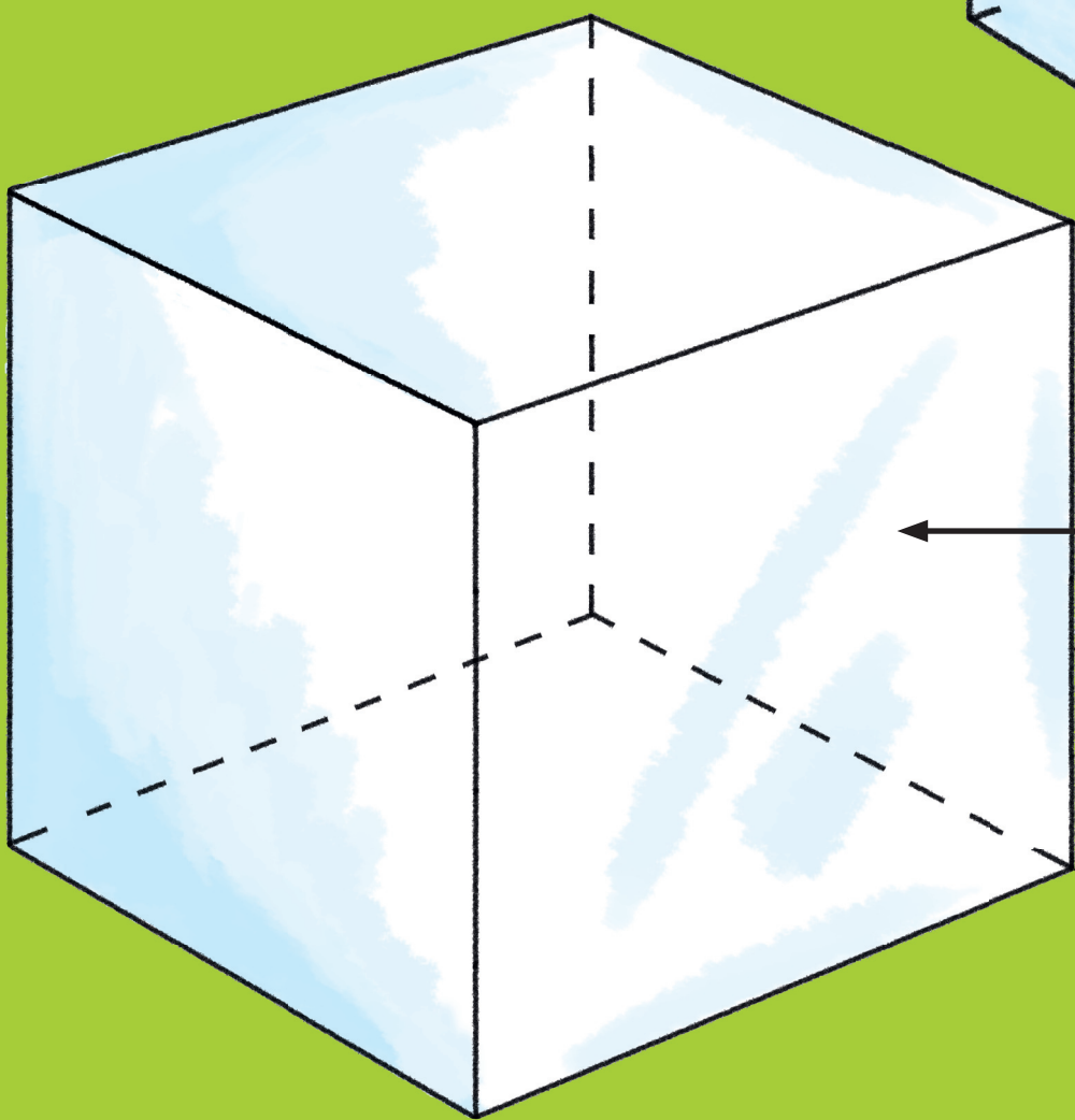
Würfel
