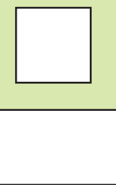
Rechteck
